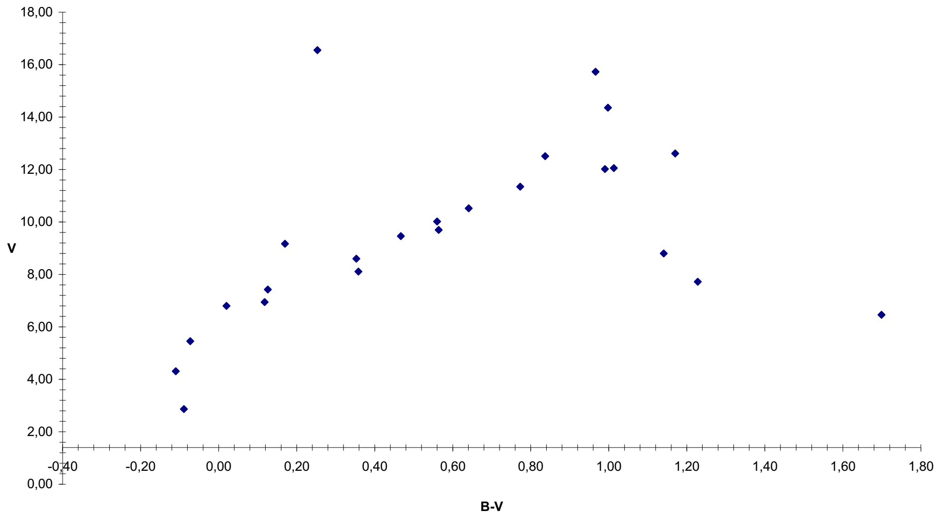
Barevný diagram I. (závislost V na B-V)
