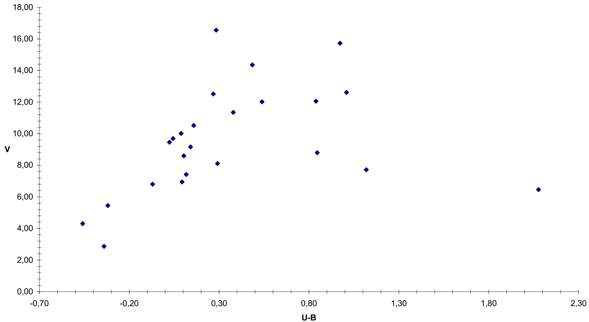
Barevný diagram III (závislost V na U-B)
